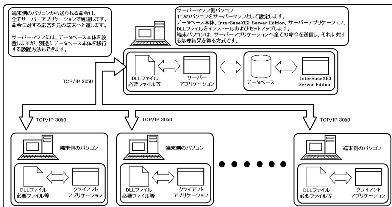
図2. ローカルネットワーク接続タイプの図解
